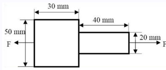
Figura 1: Pieza escalonada de sección circular sometida a tracción.
