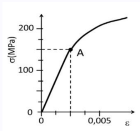
Figura 2: Diagrama tensión-deformación; el punto A marca el límite elástico.
