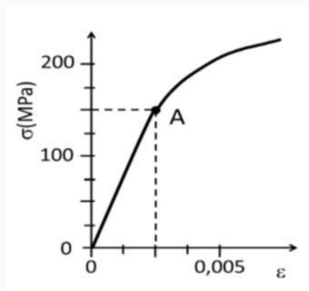
Figura 3: Diagrama tensión-deformación; el punto A marca el límite elástico.
